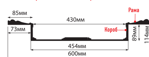
KS61A-19D рама: 600x600x25, короб: 454x454x89
