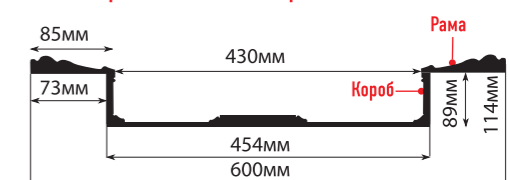
KS61A-57 рама: 600x600x25, короб: 454x454x89
